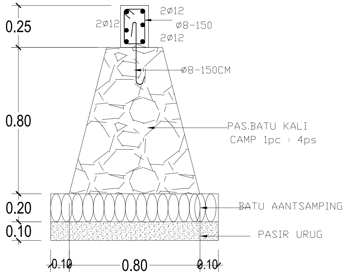
POTONGAN A-A
